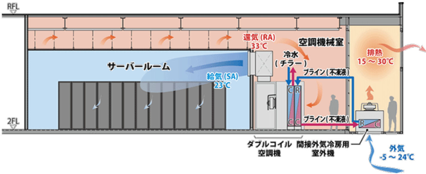
1・2号棟の運用知見を反映 冷媒を外気で冷却し、外気を直接取り込まずに冷熱を活用
