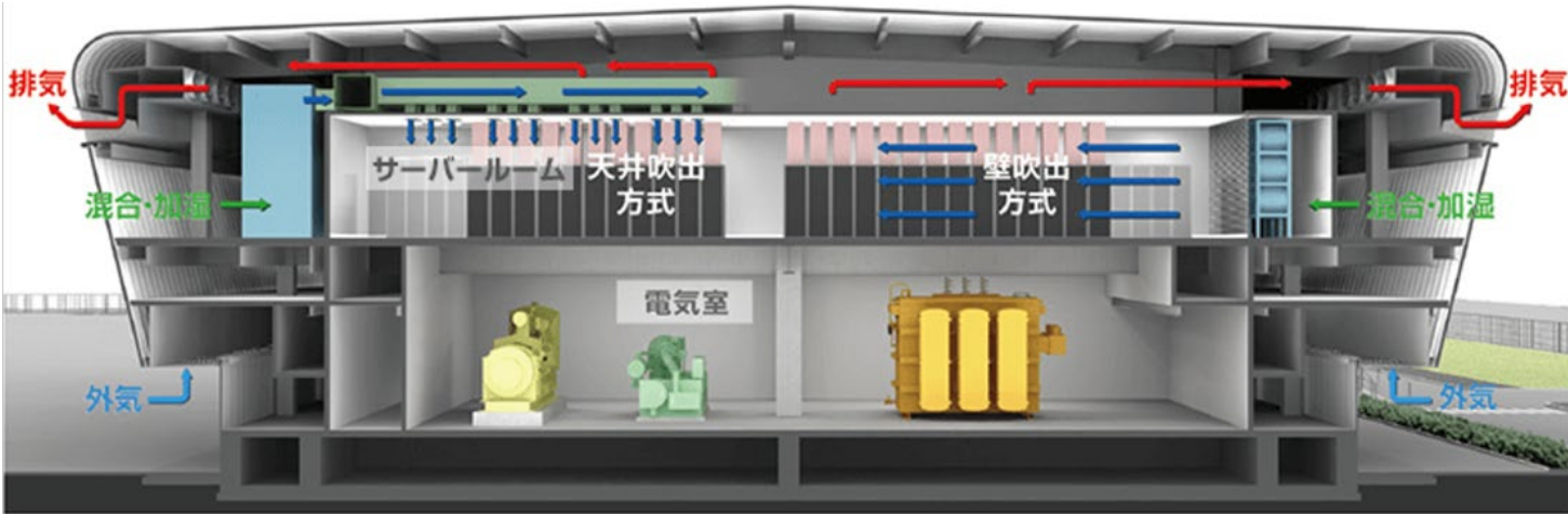
北海道の冷涼な外気を直接取り込み、サーバーの冷却に活用 モジュール設計により柔軟な拡張にも対応
