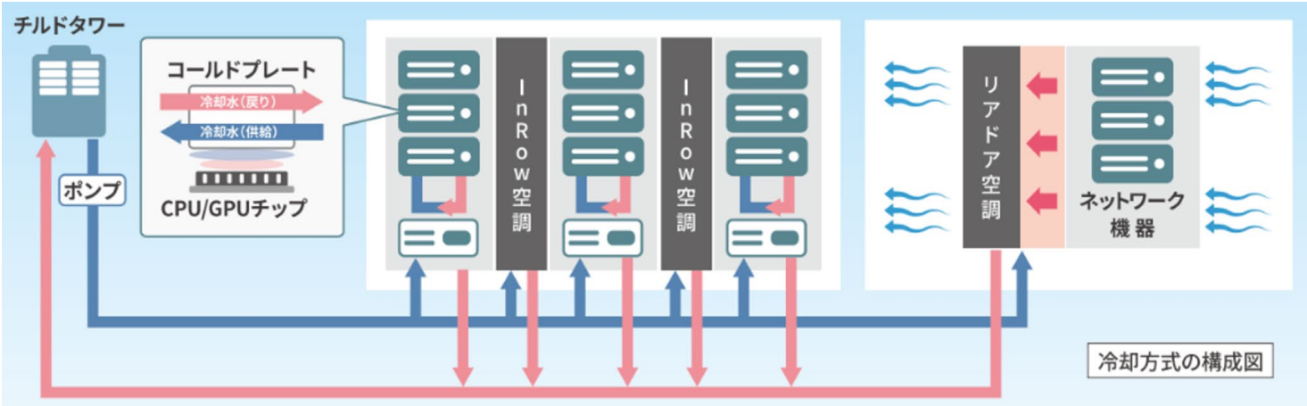
高発熱なGPUサーバーを冷却水で効率的に冷却 高密度化と迅速・柔軟な設備拡張に対応
