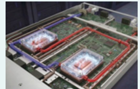
液冷2相システムの中核機器の一つであるコールドプレート (イメージ)
