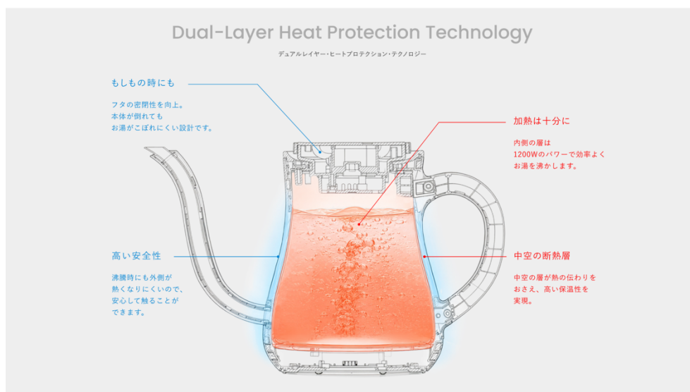
もしもの時にも安心の筐体二重構造
