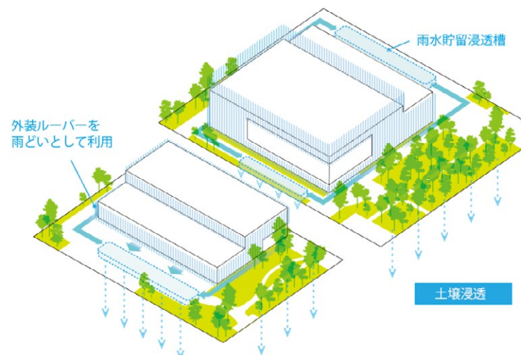
KIHにおける雨水活用と地下水涵養の仕組み
