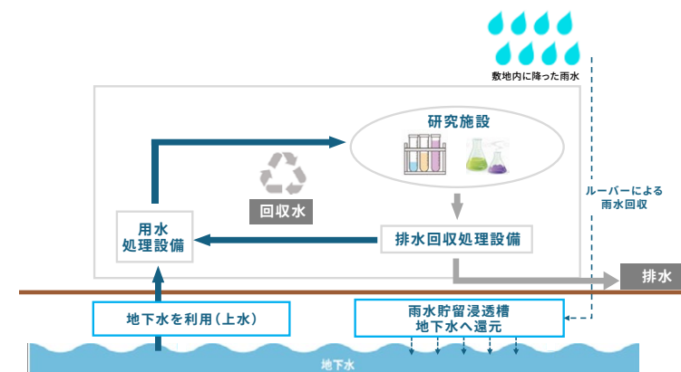
KIHにおける水循環の全体像
