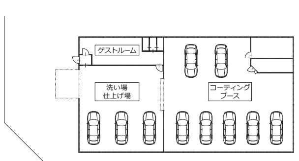
【店舗平面図】
