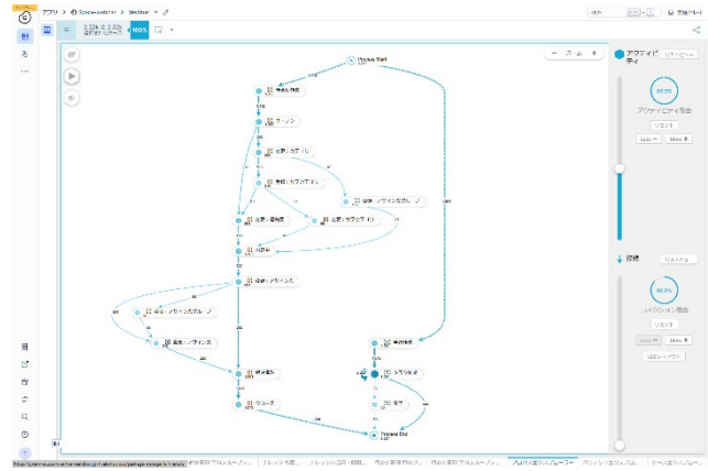
図2.プロセスエクスプローラー画面
